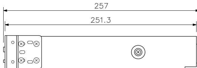
側面図
