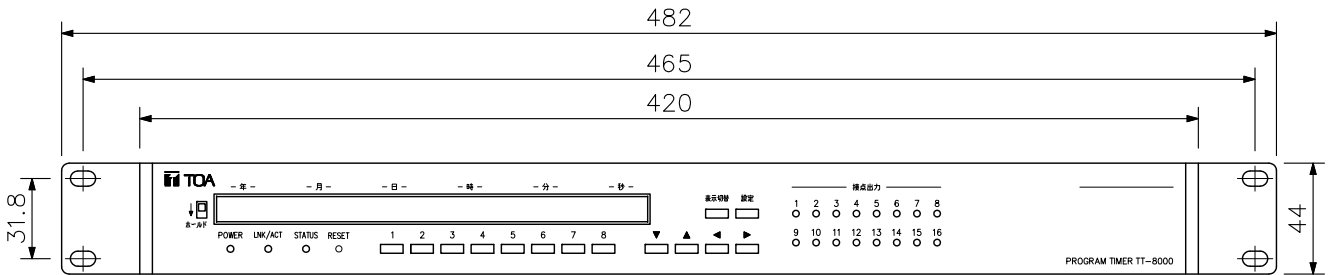
正面図
