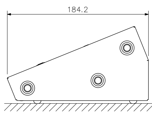
据置図
