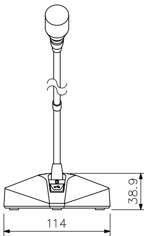
正面図
