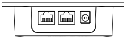
上面図
