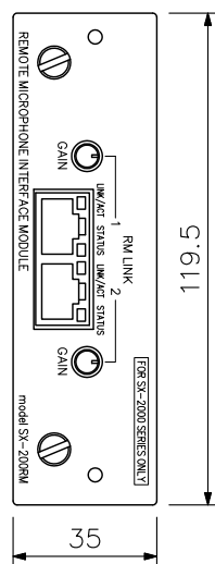
正面図
