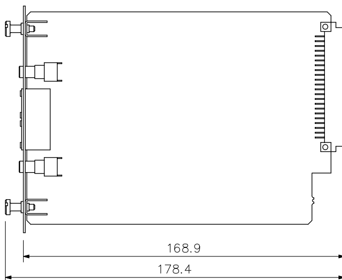
側面図
