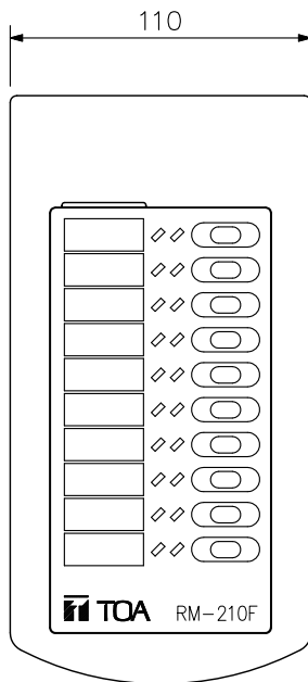
A矢視図
