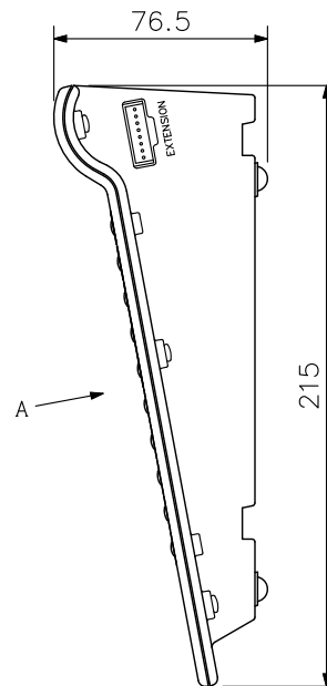
側面図
