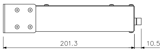
側面図
