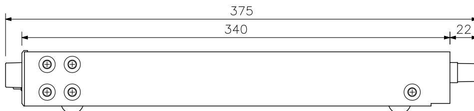
側面図
