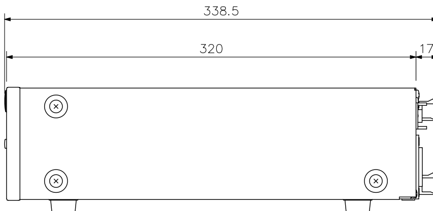
側面図
