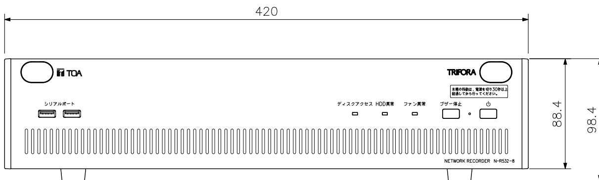
正面図
