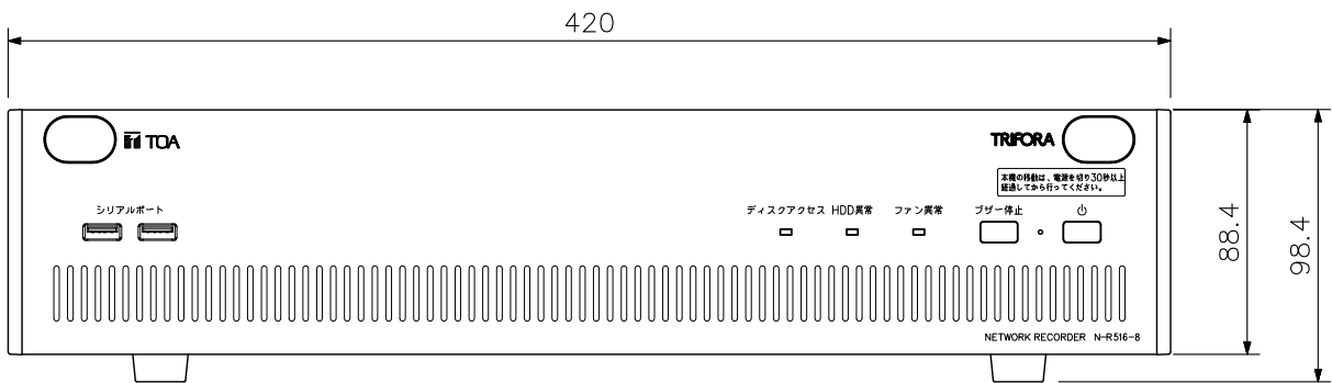
正面図
