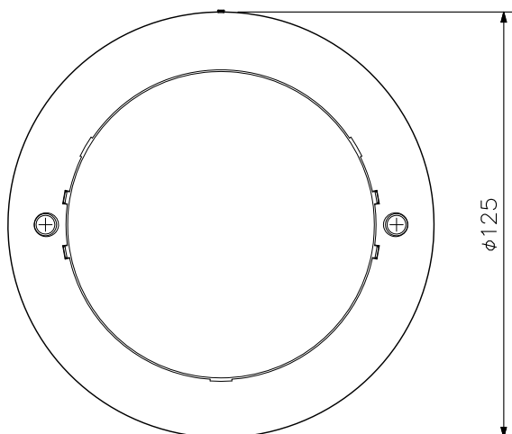
底面図
