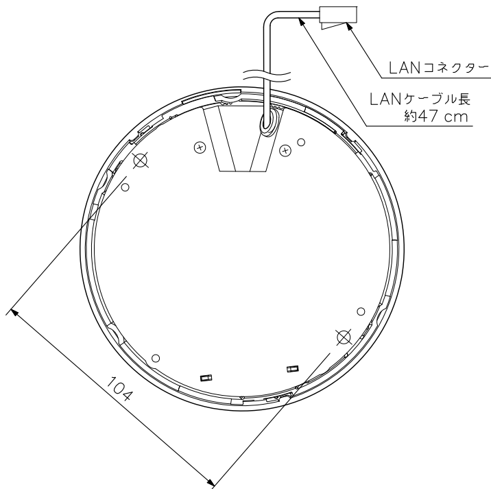
上面図
