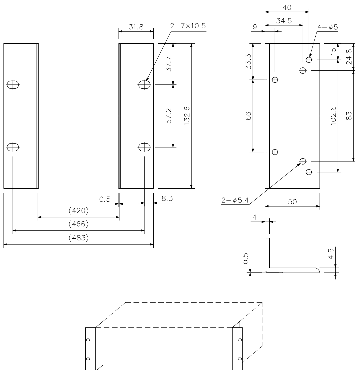
取付参考図
