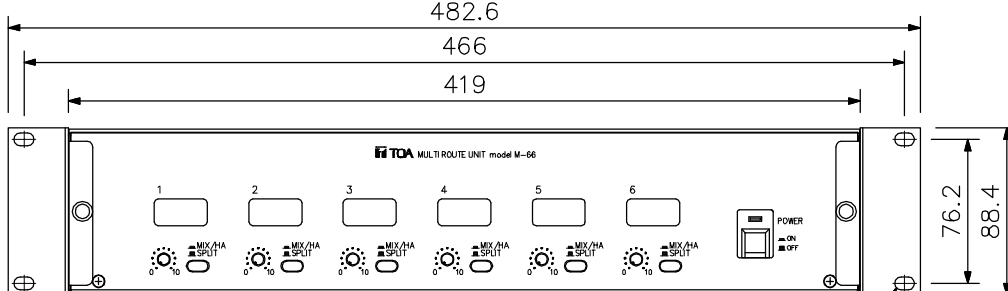
正面図
