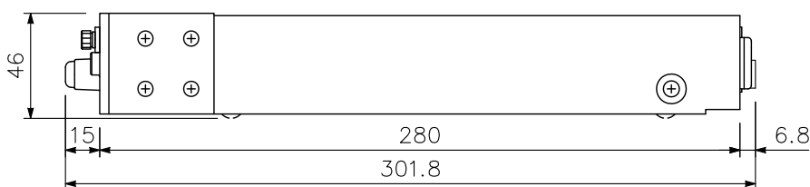
側面図
