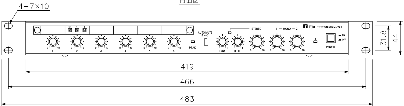
正面図
