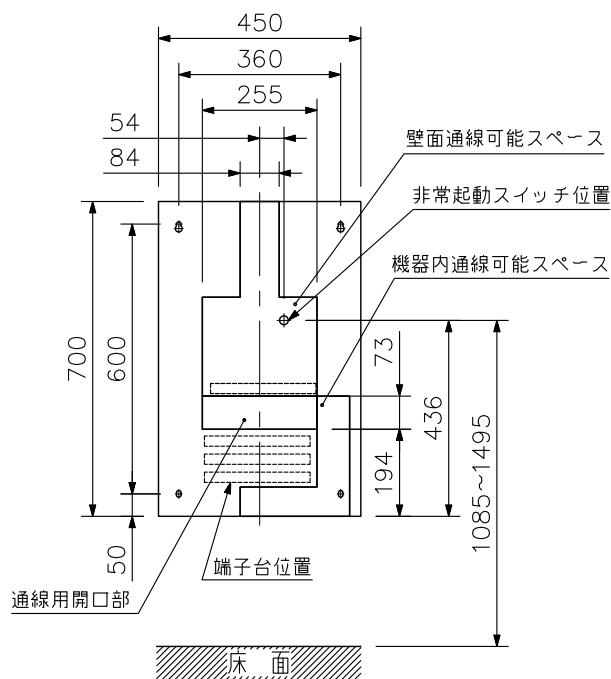
壁取付工事図
