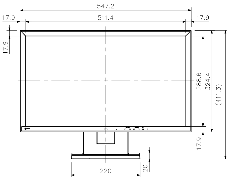
正面図
