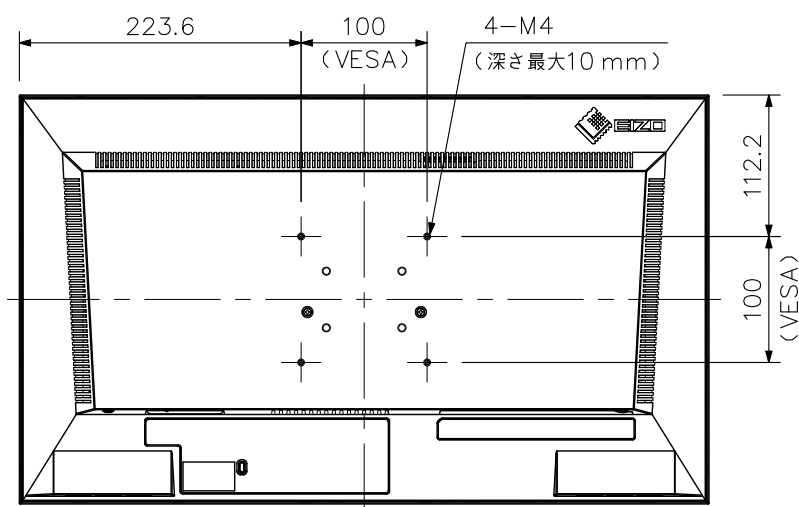
背面図
