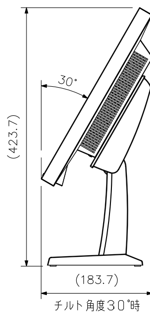
側面図
