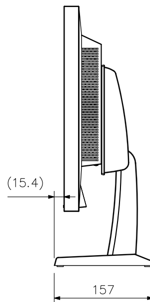
側面図
