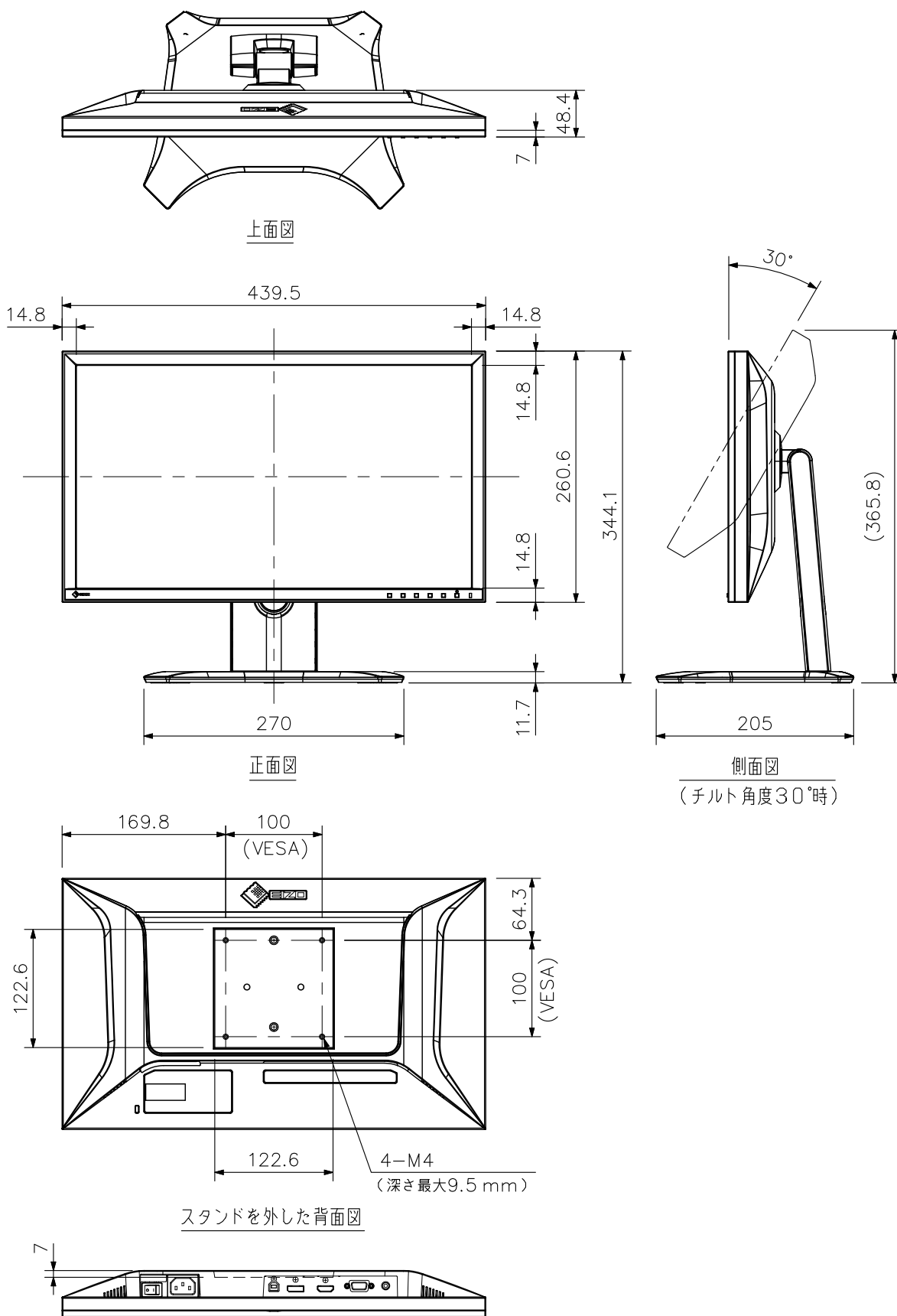
底面図
