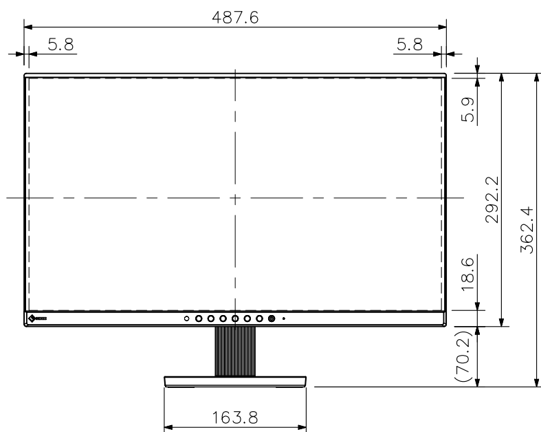
正面図
