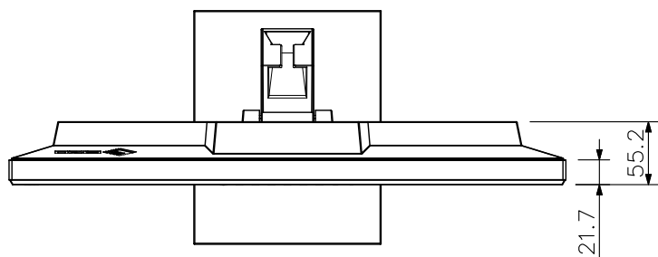
上面図
