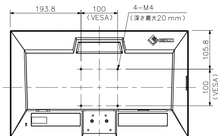
背面図
