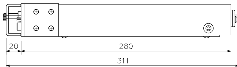
側面図
