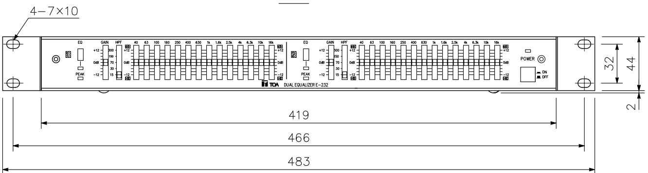
正面図
