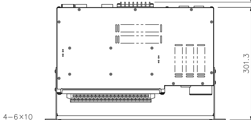
上面図
