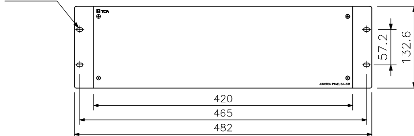
正面図
