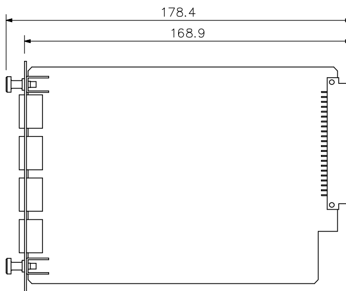
側面図
