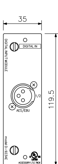
正面図
