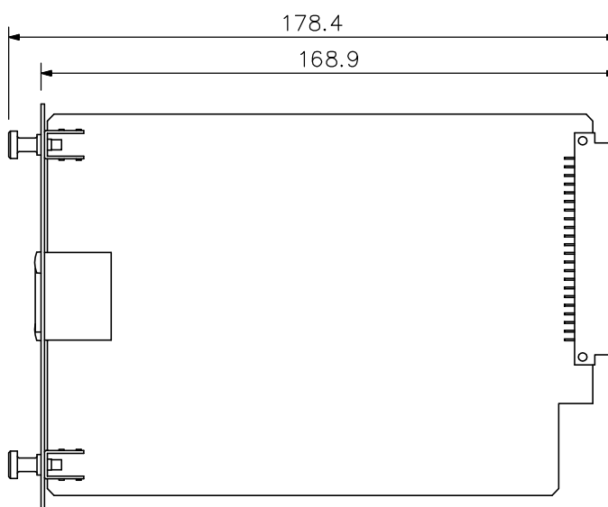
側面図
