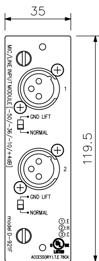
正面図
