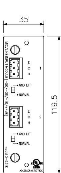
正面図
