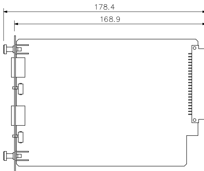
側面図
