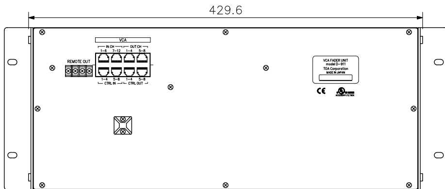
背面図
