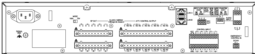
背面図
