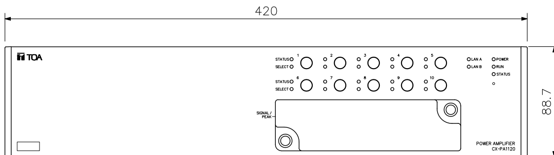
正面図
