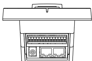
底面図
