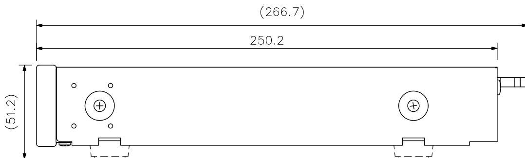
側面図
