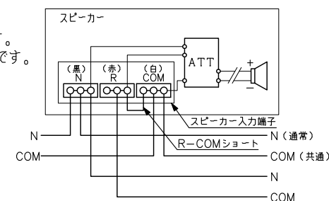
結線図
