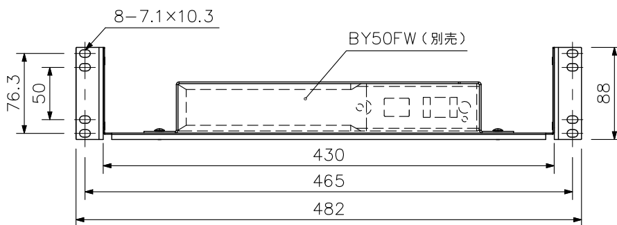
正面図
