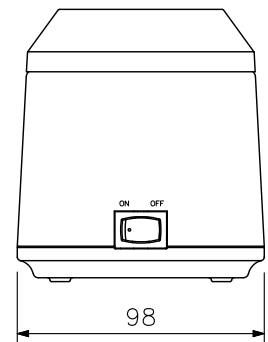
右側面図
