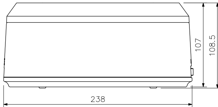
正面図
