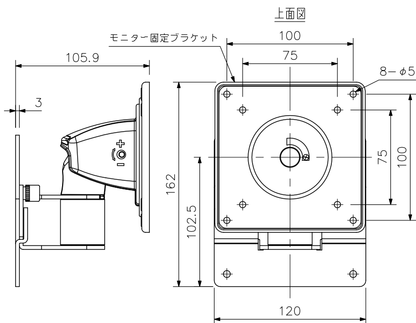
側面図
