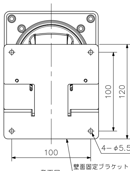
背面図
