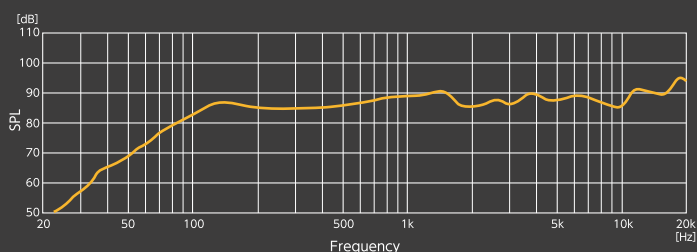
SR-F04 | 周波数特性グラフ
