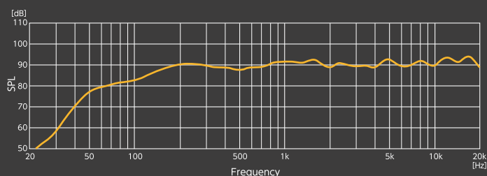
SR-F08 | 周波数特性グラフ
