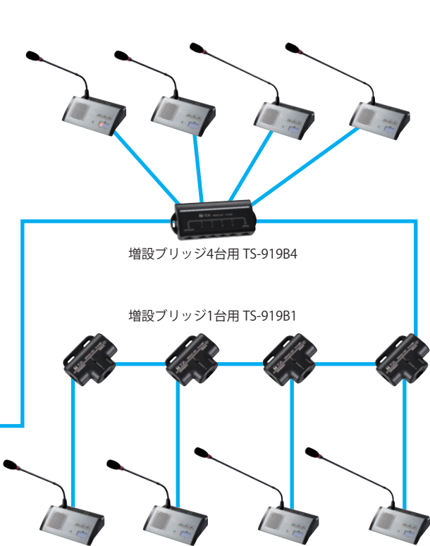
有線会議ユニット TS-911／912／811／812
